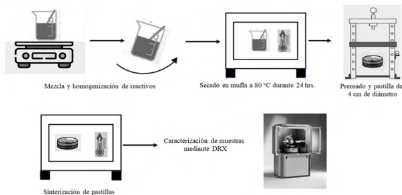
Figura 1. Esquema de la metodología de síntesis de pastillas cerámicas.
