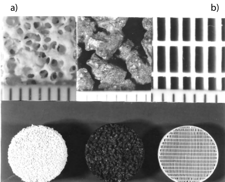
Figura 2. Fotografías de a) filtros FICELEP y b) espumas cerámicas. Las fotografías superiores muestran el plano de entrada de fluido al interior de los filtros, mientras que las fotografías inferiores representan una vista de una sección longitudinal de los filtros, es decir un corte a lo largo del espesor de las piezas. Referencia [1].
