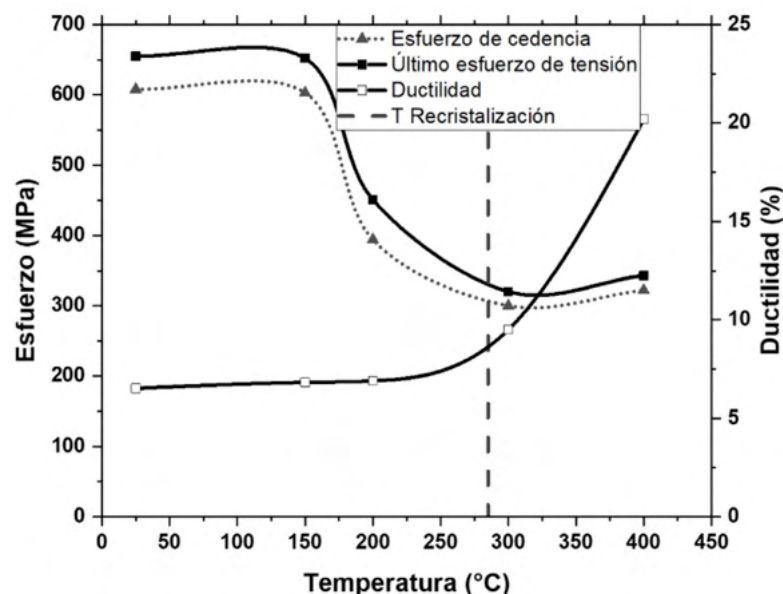
Fig. 3. Estabilidad térmica de las propiedades mecánicas de la aleación procesada por ARB y T6.
