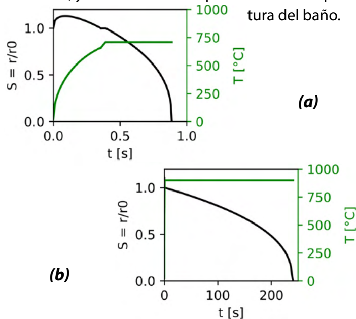
Figura 2. Perfil de posición adimensional de la interfase y de la temperatura de la adición para, (a) adición del Grupo I (Al-20%Si), (b) adición del Grupo II (Si puro), en un baño a 900°C, y con diámetro inicial de 2.5 cm.
