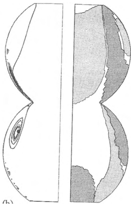
Figura 3. Sección izquierda: trayectoria calculada de partículas suspendidas en aluminio fundido y atrapadas en las paredes de un filtro. Sección derecha: Las zonas de color gris representan regiones donde la velocidad del líquido cambia como resultado de la obstrucción provocada por las partículas atrapadas. Referencia [1].
