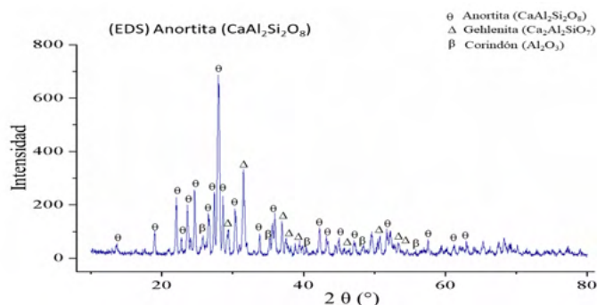
Figura 4. Patrón de difracción para el compuesto anortita ( \text{CaAl}_2\text{Si}_2\text{O}_8 ) obtenido a partir de escoria de aluminio.
