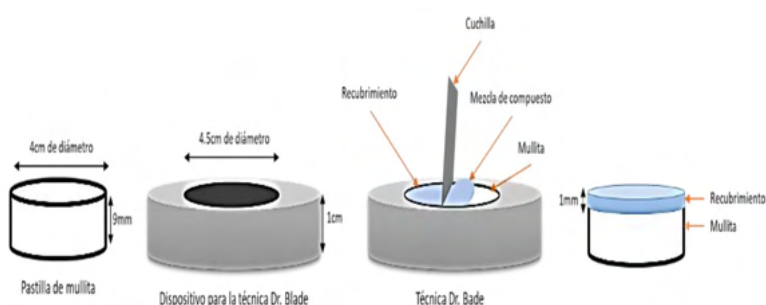
Figura 2. Técnica Dr. Blade para recubrimientos [5].
