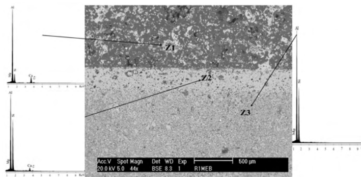
Figura 5. Micrografía por MEB del compuesto anortita ( \text{CaAl}_2\text{Si}_2\text{O}_8 ) con prueba de corrosión.
