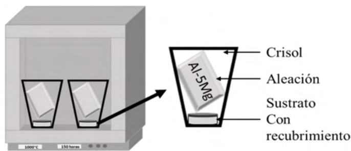
Figura 3. Esquema de la prueba de corrosión.
