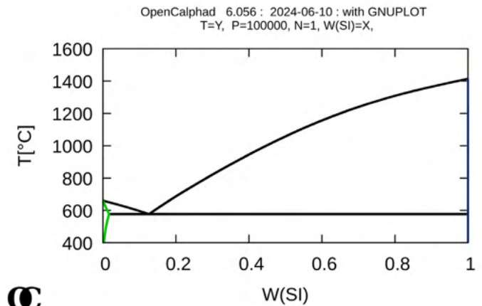
Figura 1. Diagrama binario Aluminio-Silicio. El eje vertical indica la temperatura en °C, y el horizontal la fracción másica de silicio.
